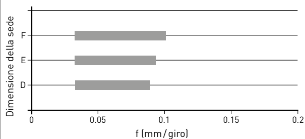
Rompitruciolo R08-GS
