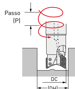
2.2 Fori passanti
