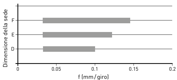
Rompitruciolo R/L05-GM
